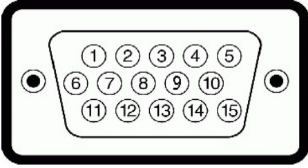
핀 번호 모니터 쪽의 15핀 신호 케이블
