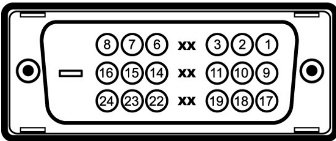
핀 번호 모니터 쪽의 24 핀 신호 케이블
